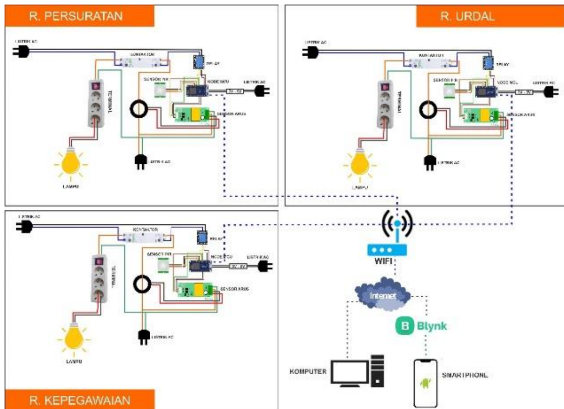
Gambar 3. Rancangan Sistem Ruang yang dikontrol
