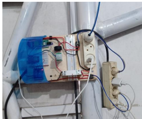
Gambar 5. Rancangan Alat untuk Ruang Persuratan
