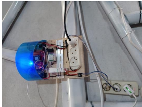
Gambar 4. Rancangan Alat untuk Ruang Kepegawaian
