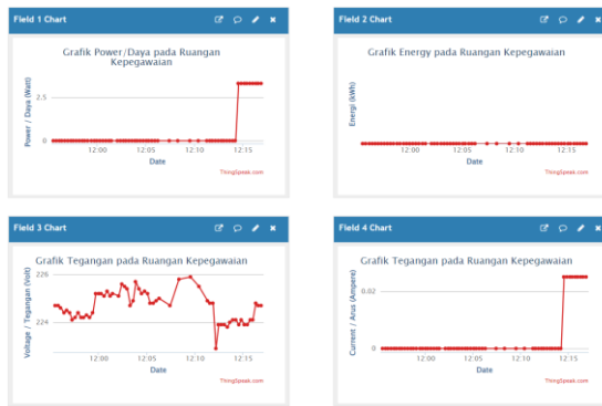
Gambar 10. Grafik Komsumsi Listrik Ruang Kepegawaian
