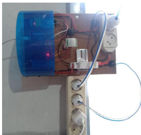
Gambar 6. Rancangan Alat Mikronroller untuk Ruang Urdal
